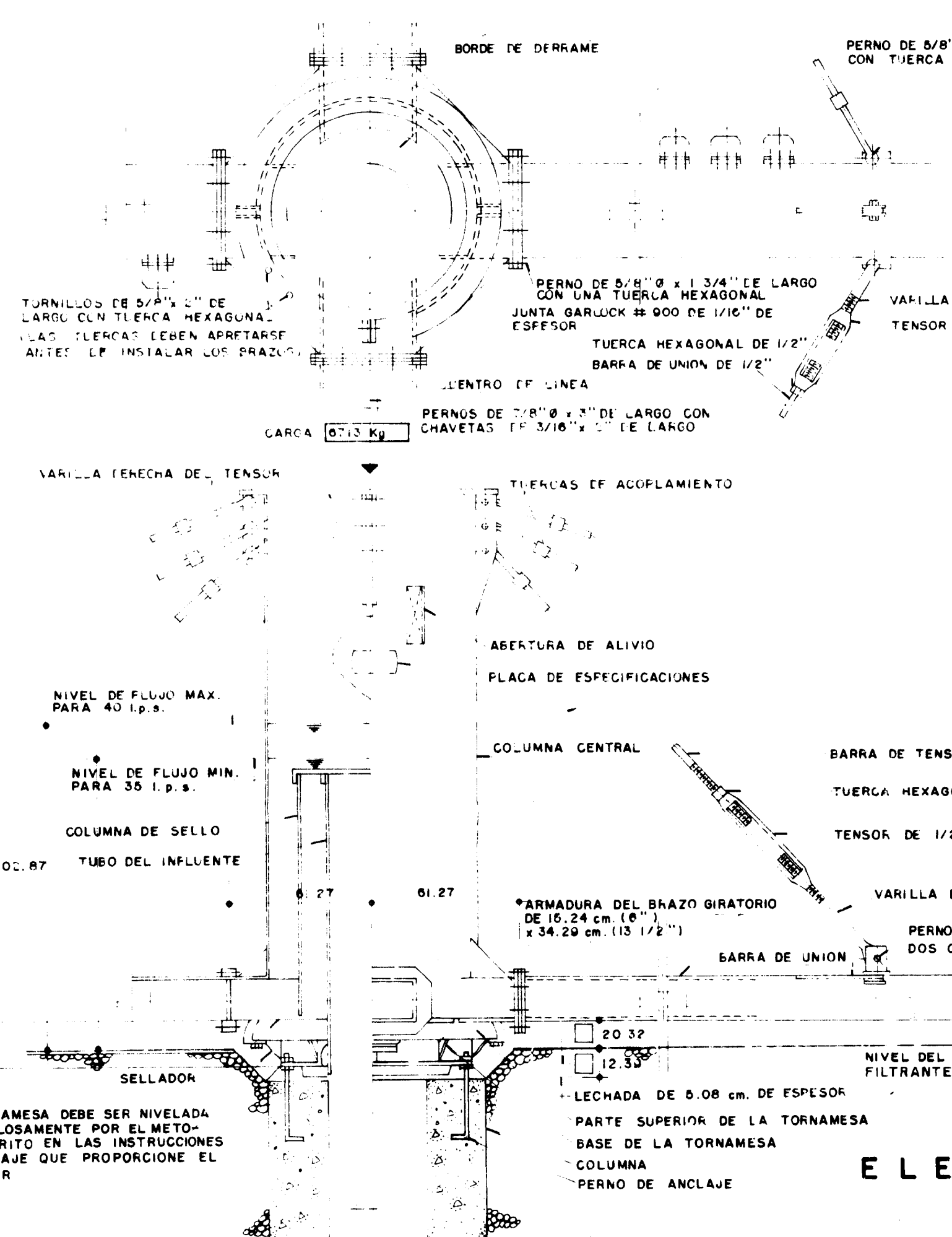
PERFIL CENTRO DEL TANQUE DE SEDIMENTACION PRIMARIA DETALLE - 3
