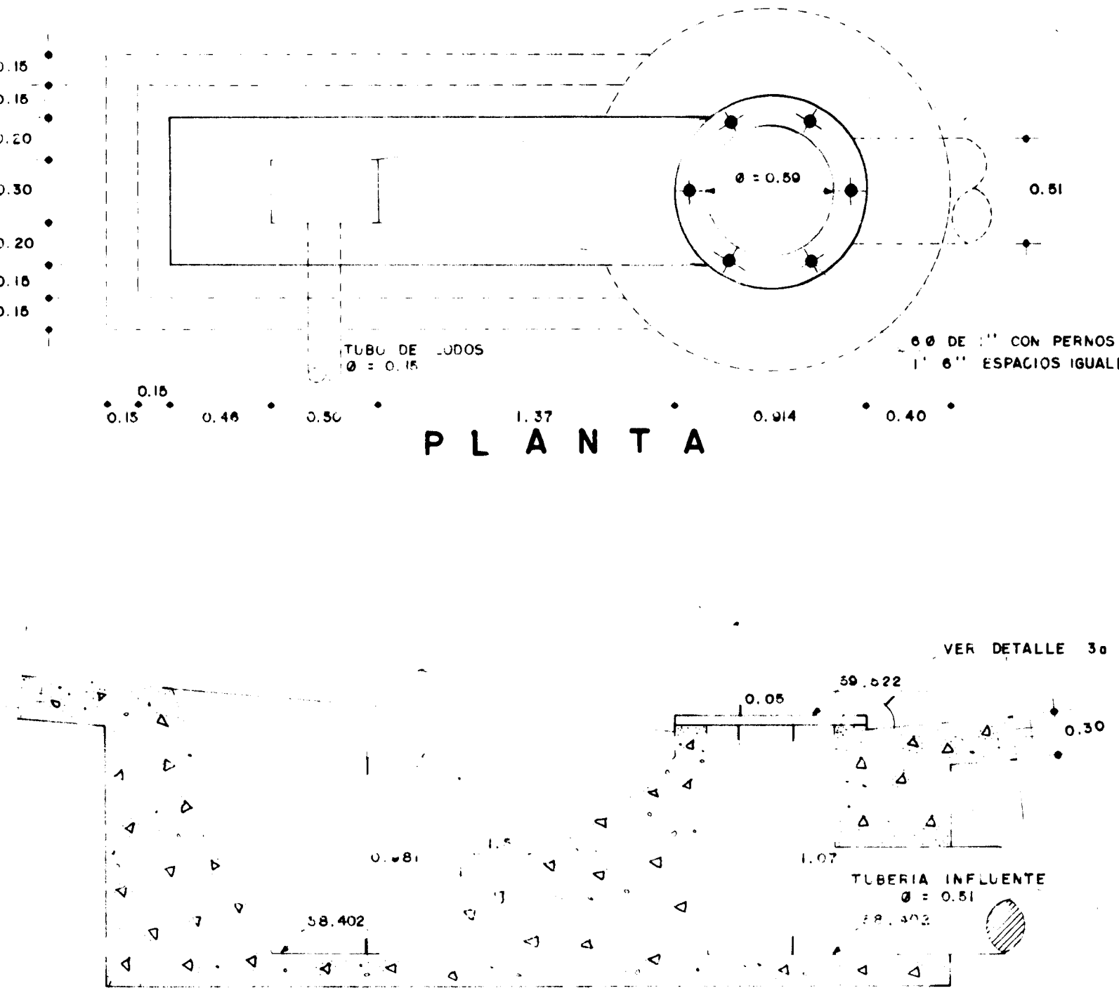
PERFIL CENTRO DEL TANQUE DE SEDIMENTACION PRIMARIA DETALLE - 3
