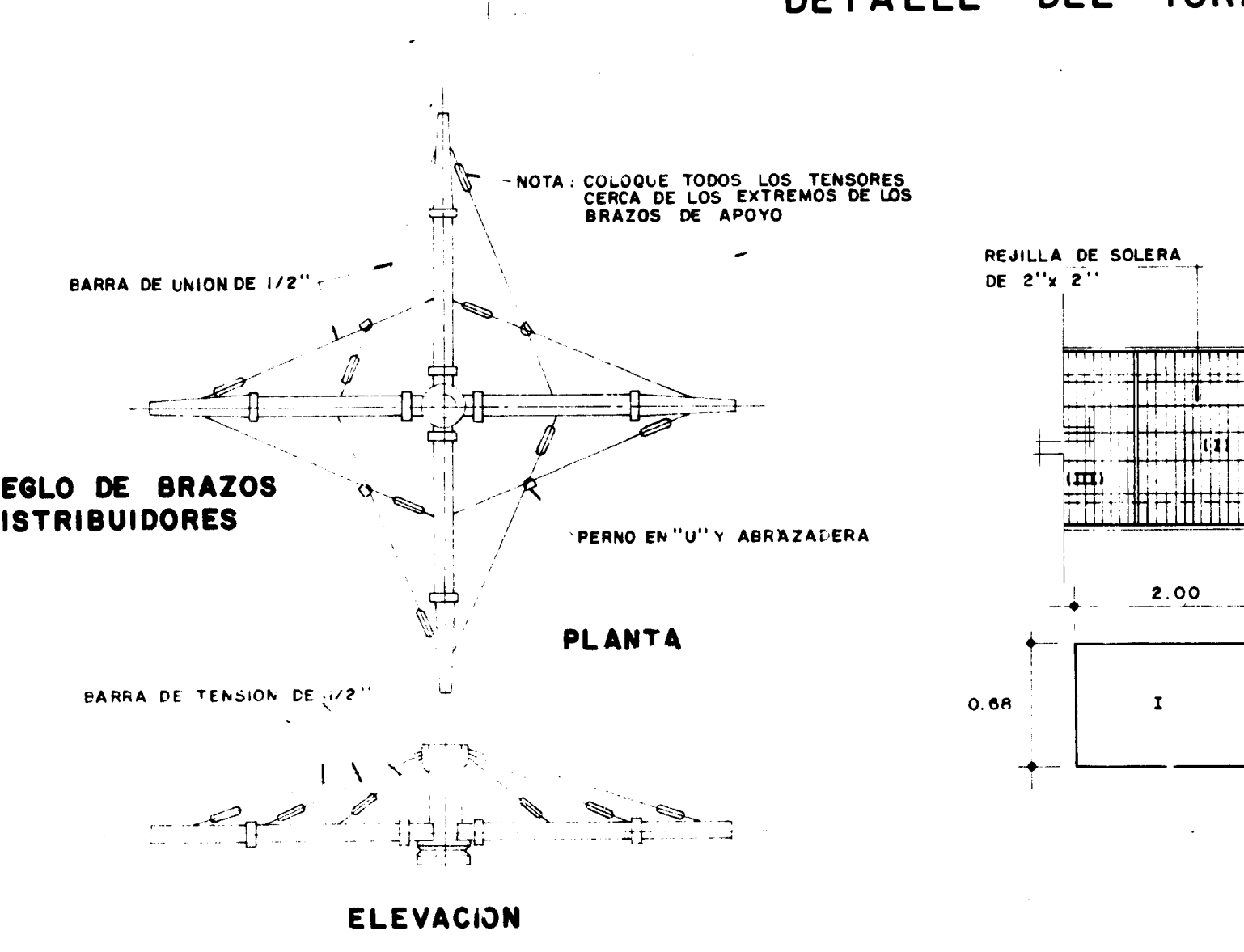
ARREGLO DE BRAZOS DISTRIBUIDORES
