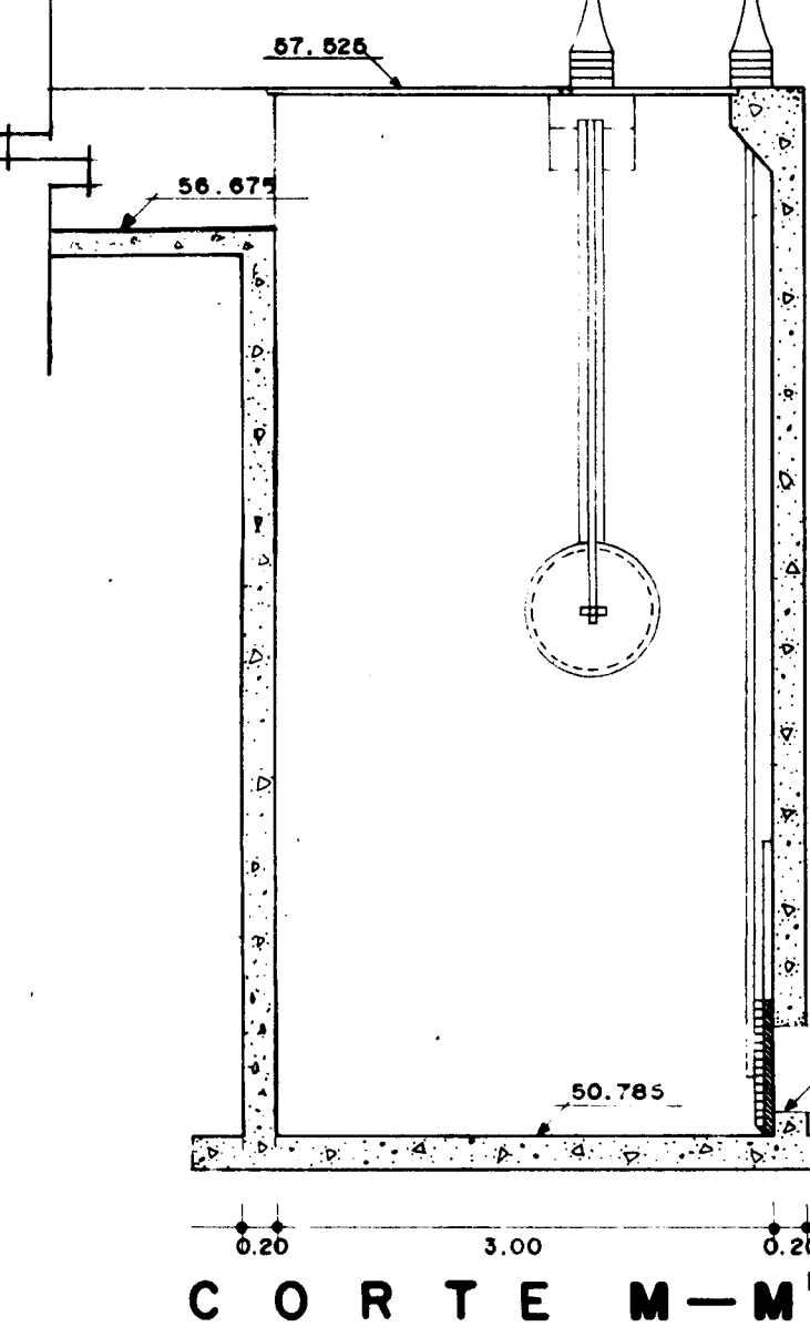
CORTE M-M'
