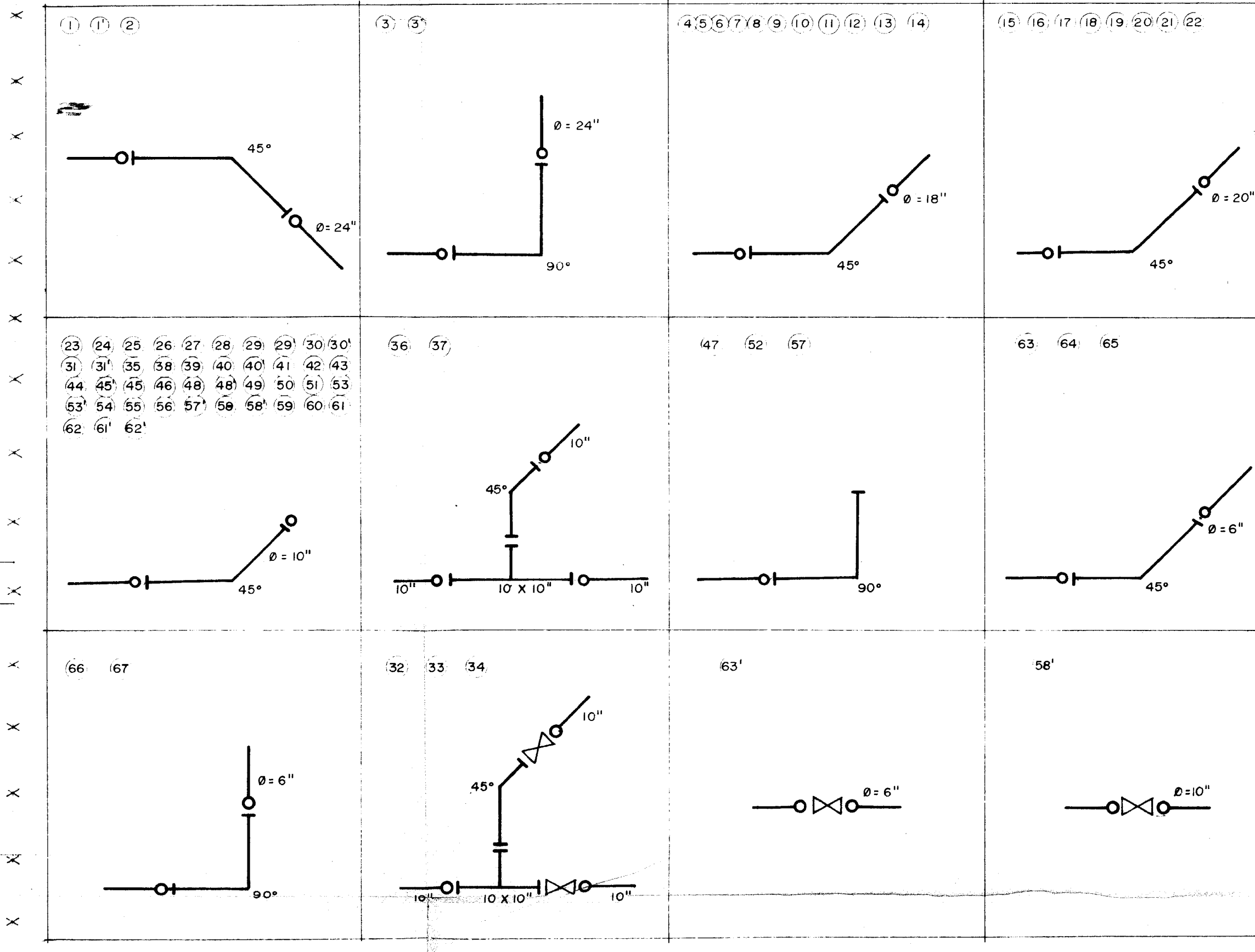
CRUCEROS DE LAS LINEAS DE INTERCONEXION
