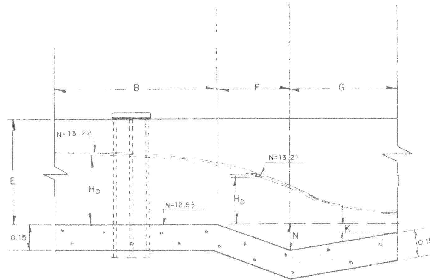
CCORTE A-A
